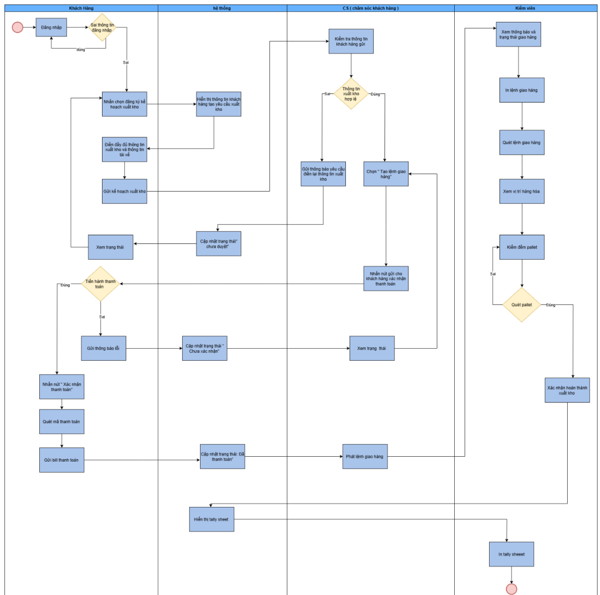
Hình 2.1: Workflow hệ thống xuất kho
