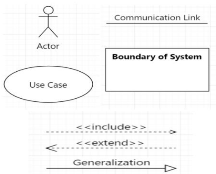
Hình 1.5: Các thành phần cơ bản của use case. Nguồn [6]
