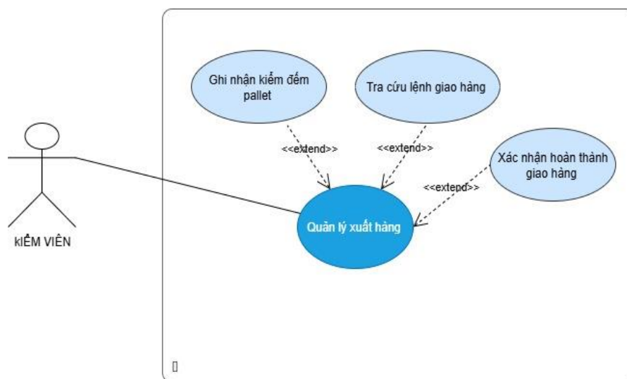
Hình 2.6: Use case của tác nhân kiểm viên
