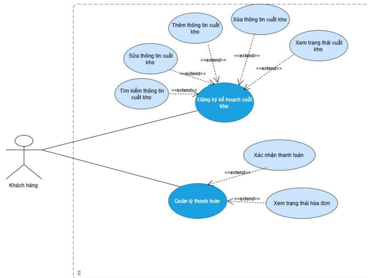
Hình 2.4: Use case của tác nhân khách hàng
