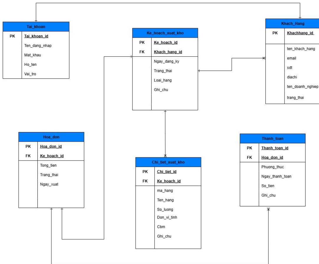
Hình 3.1: Sơ đồ quan hệ của các bảng
