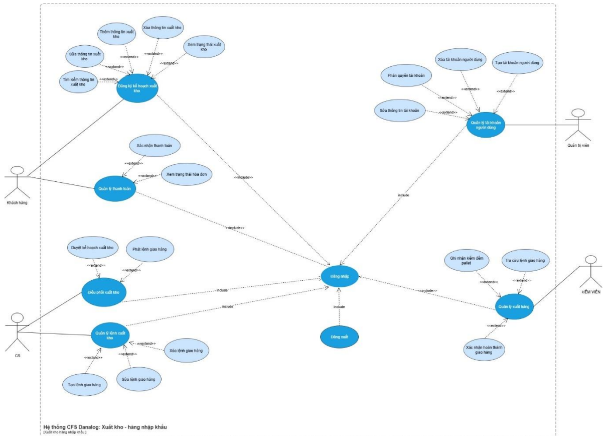
Hình 2.2: Use case tổng quát của hệ thống
