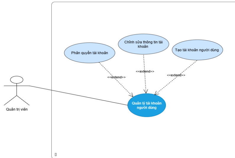
Hình 2.3: Use case của tác nhân quản trị viên
