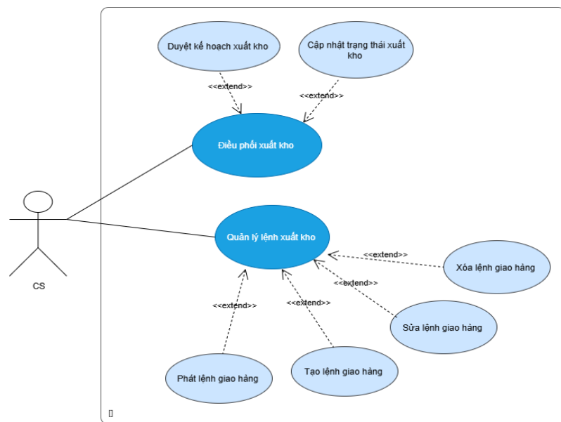
Hình 2.5: Use case của tác nhân CS
